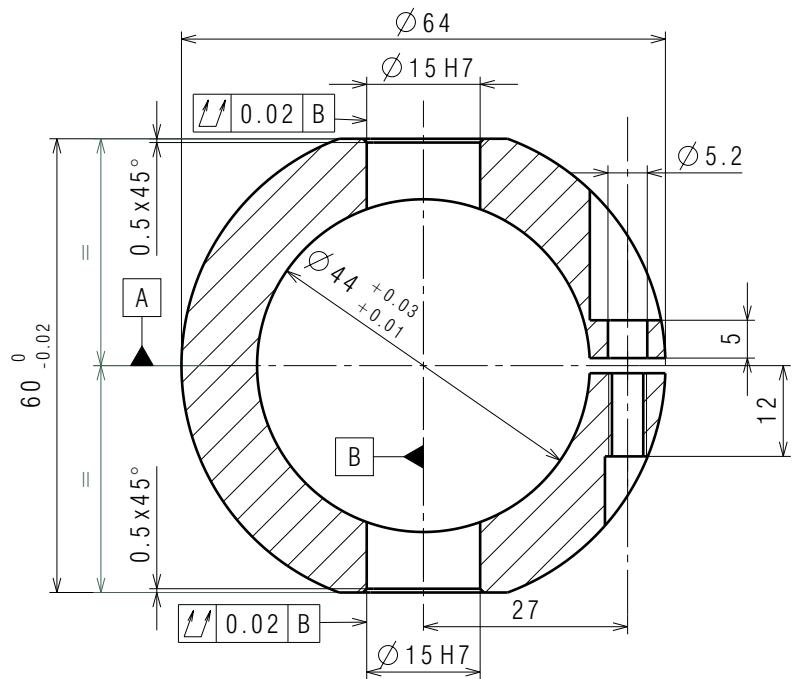
Schnitt A-A
