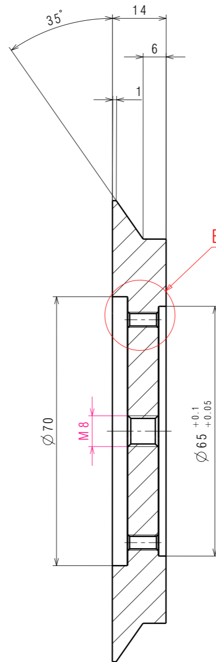
Cut A-A
