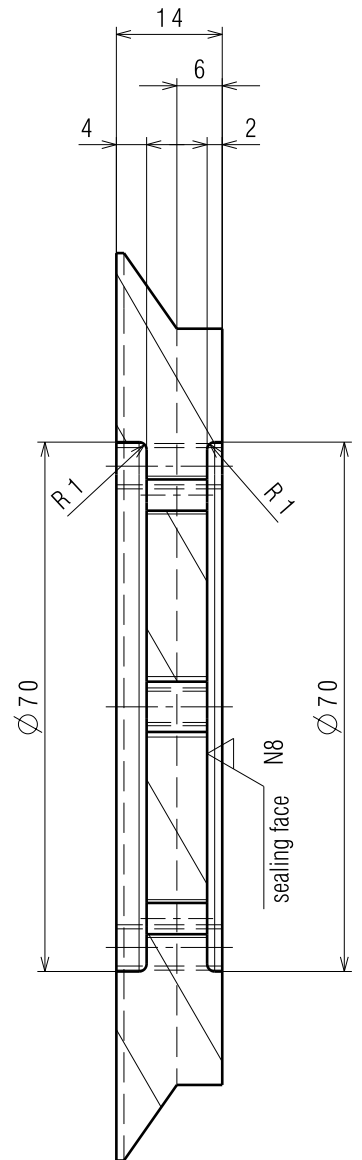
Cut A-A
